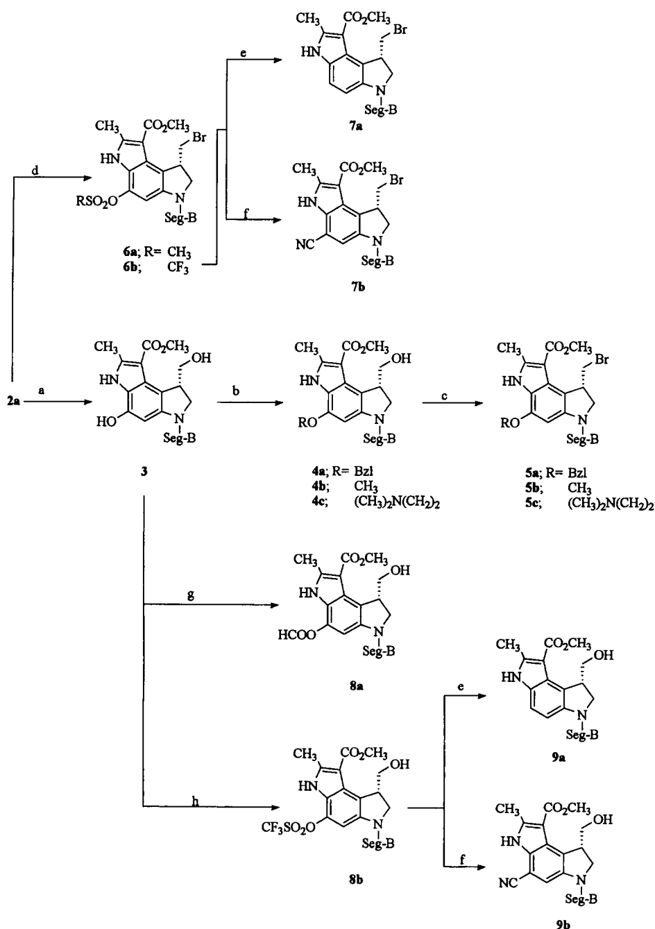
Scheme 1. (a) 70% HClO 4 , DMF; (b) BzlBr or CH 3 I or N,N -dimethylaminoethyl chloride, K 2 CO 3 , DMF; (c) MsCl, pyridine, then LiBr, DMF; or CBr 4 , PPh 3 , CH 2 Cl 2 ; (d) HBr, CH 3 CN, then CH 3 SO 2 Cl or (CF 3 SO 2 ) 2 O, Et 3 N, CH 2 Cl 2 ; (e) Pd(OAc) 2 , 1,1'-bis(diphenylphosphino)ferrocene, Et 3 N, HCOOH, DMF; (f) n -Bu 3 SnCN, (PPh 3 ) 4 Pd, CH 2 Cl 2 ; (g) (CF 3 SO 2 ) 2 O, Et 3 N, DMF; (h) (CF 3 SO 2 ) 2 NPh, Et 3 N, DMF.
